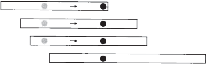
图 8-8 贪心策略
