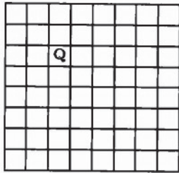
(a) 皇后的攻击范围
