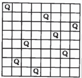
(b) 一个可行解
