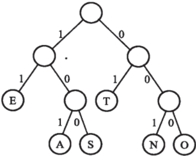
图 8-10 前缀码的二叉树表示
